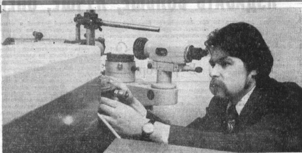
Инженер С. Ф. Старовойтов (кафедра ТОДП) проводит измерение комплексного показателя преломления диэлектрических покрытий. Фото З. Степановой.
