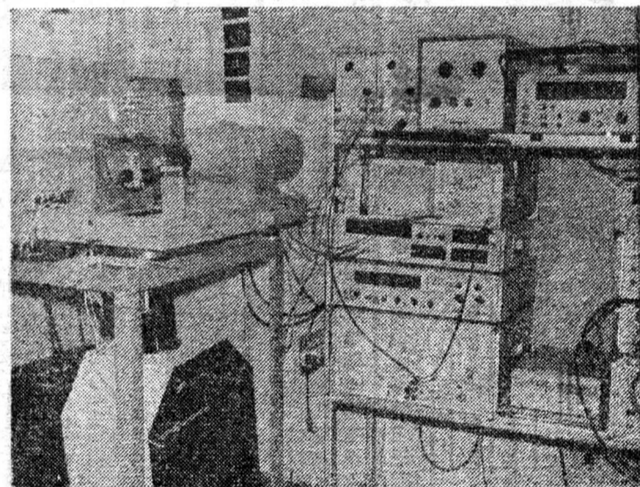
В одной из лабораторий АКОП. Стенд для исследования фотоэлектрической системы стабилизации изображения. Фото В. СОЛОВЬЕВОЙ.
